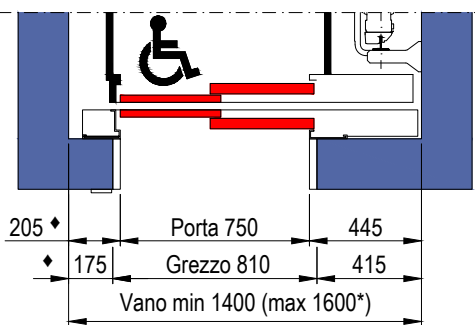
PIANTA VANO CORSA PORTE SENZA TELAIIO (E1120)
