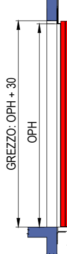
SEZIONE PORTE SENZA TELAIO (E1120)
