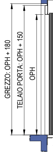
SEZIONE PORTE SENZA TELAIIO (E1120)
