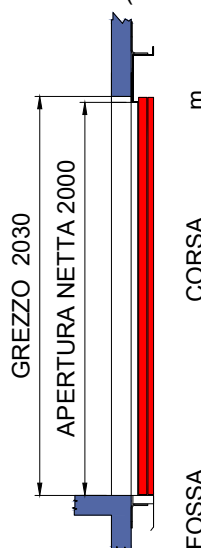
SEZIONE TELAI PORTE NF (E120)
